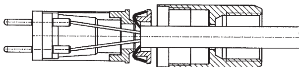
Przylutować przewody, zmontować tuleje dystansową obciąć nadmiar ekranu
